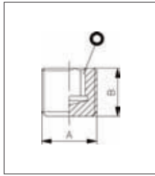
Zátka DIN 906 Male plug DIN 906
